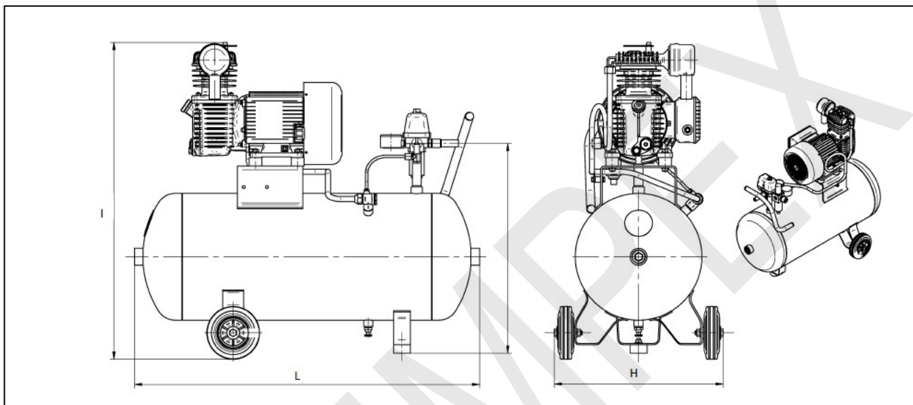
Fig. 1 Compresor cu piston:
